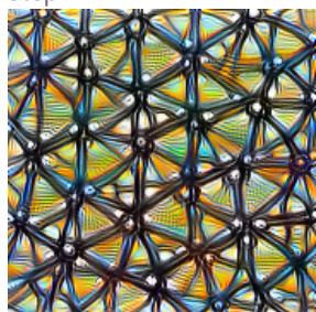
Step 2048
