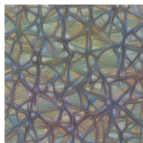
Step 48
